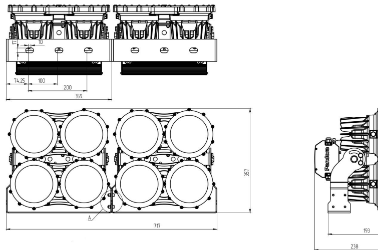
Рисунок 1. Габаритный чертеж
